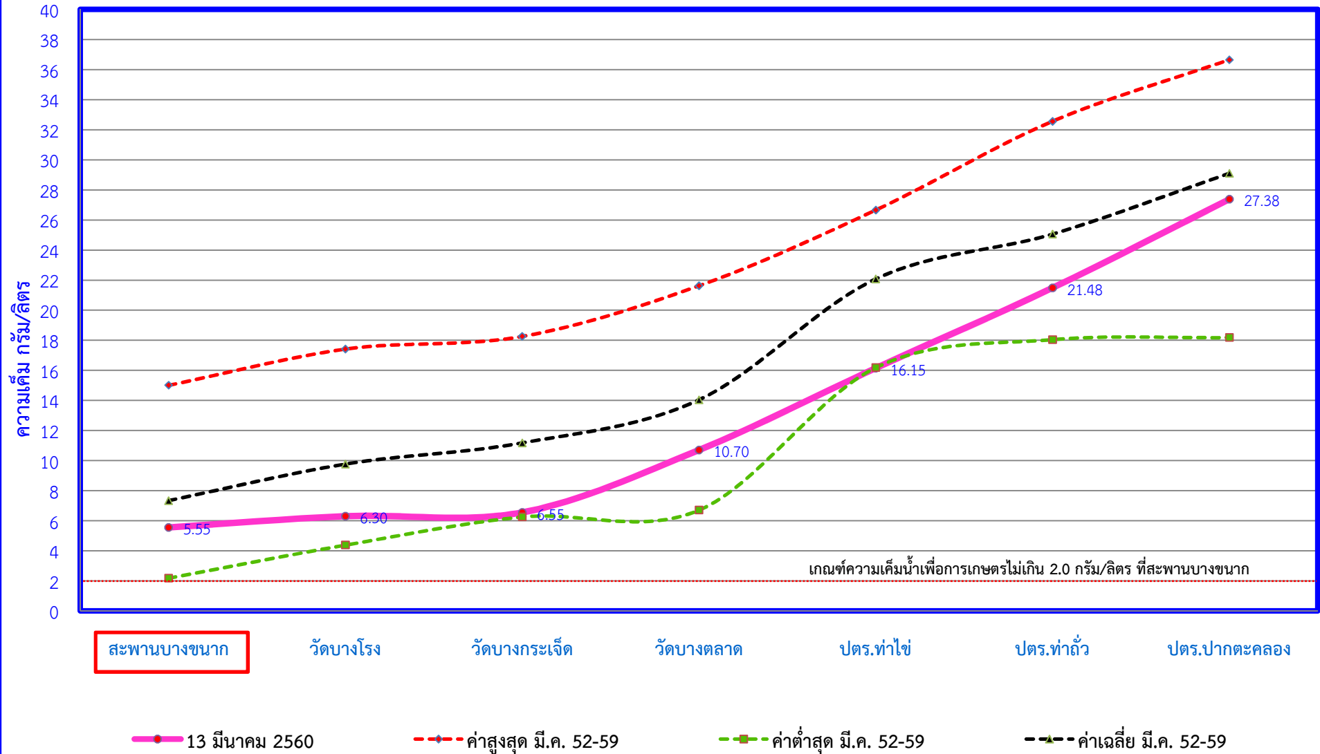
ค่าความเค็มในแม่น้ำบางปะกง วันที่ 13 มีนาคม พ.ศ. 2560
